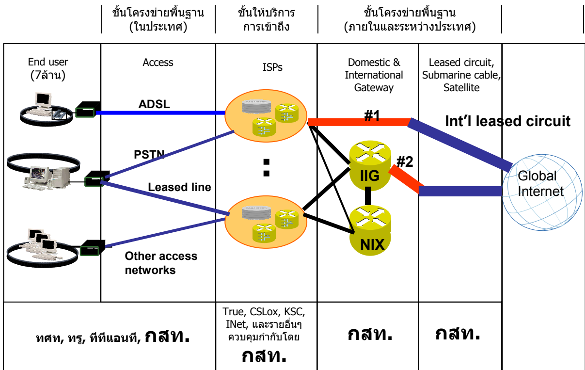
แผนภาพที่ 4.10 : ชั้นทางเทคโนโลยีของระบบอินเทอร์เน็ต (ข้อมูลเดือนเมษายน 2549)
